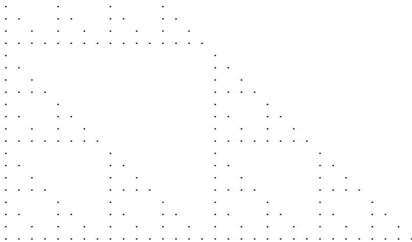
The Sierpinski-Pascal or binomial triangle
